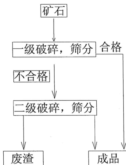
图 破碎工艺流程图
